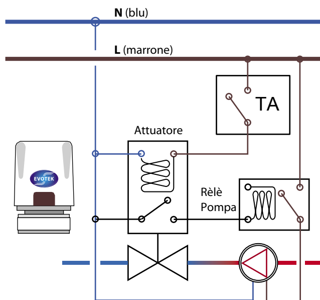
Attuatori elettrotermici con microswitch normalmente chiusi.
